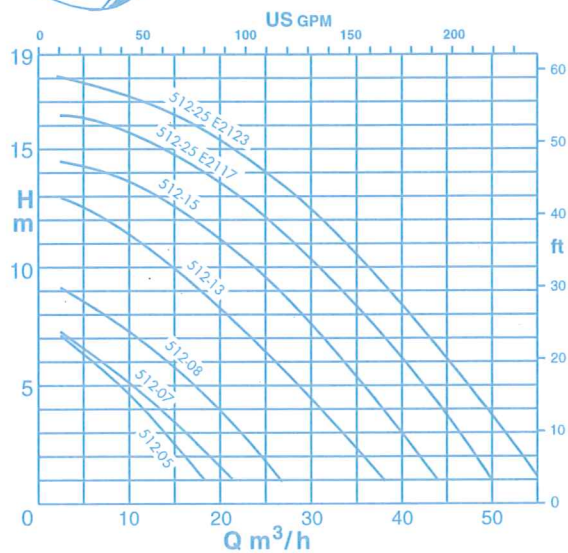
Modèle 1000 Litres
